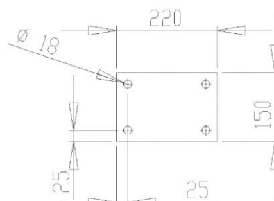
Footprint of securing plate Détail platine de pied
